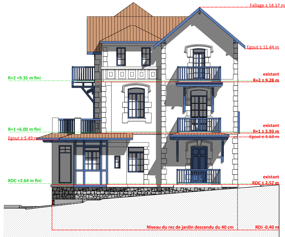
FACADE SUD - PROJET
