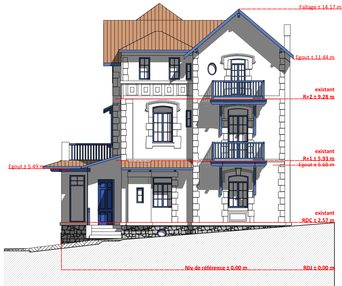
FACADE SUD - ETAT DES LIEUX
