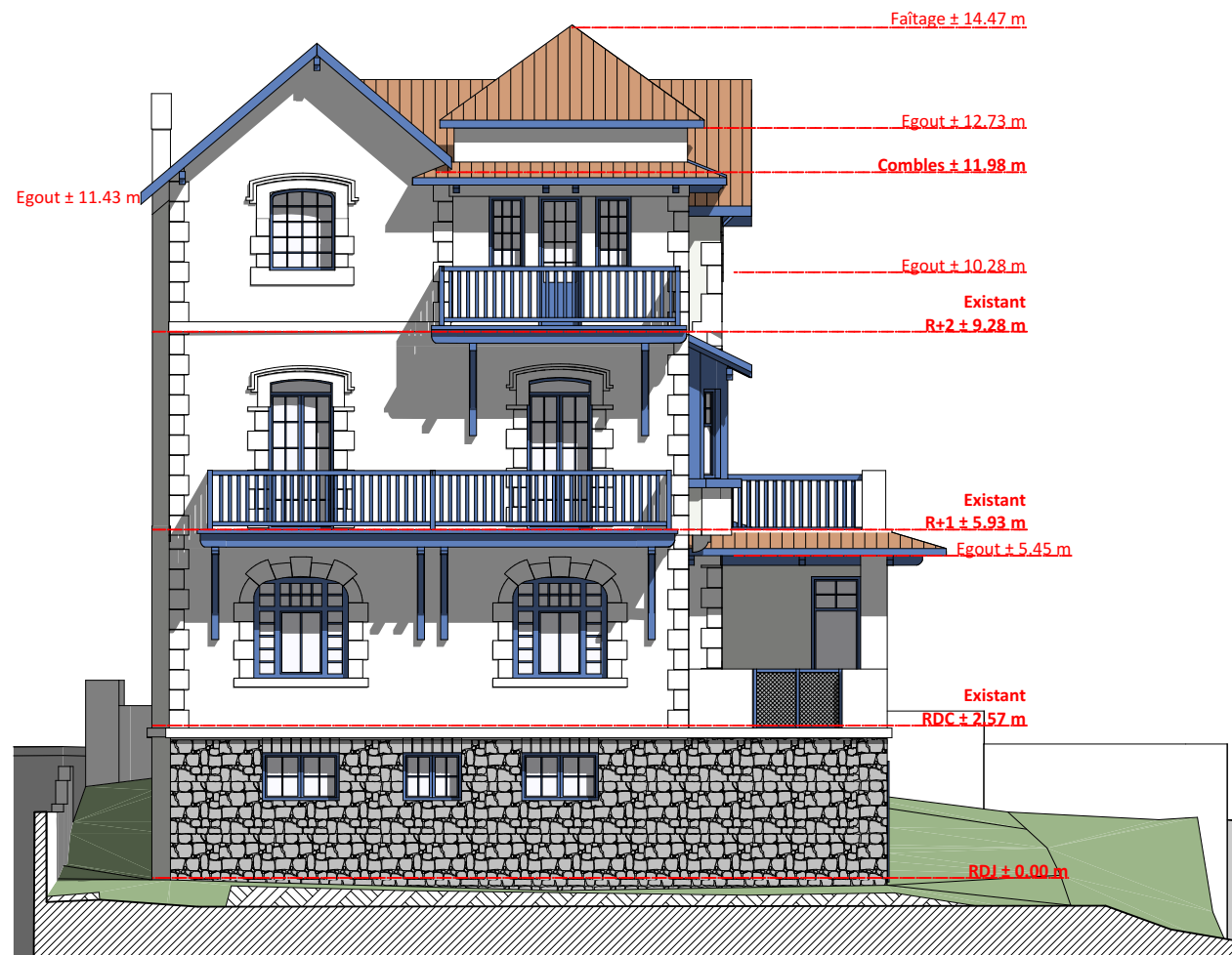
FACADE NORD - ETAT DES LIEUX
