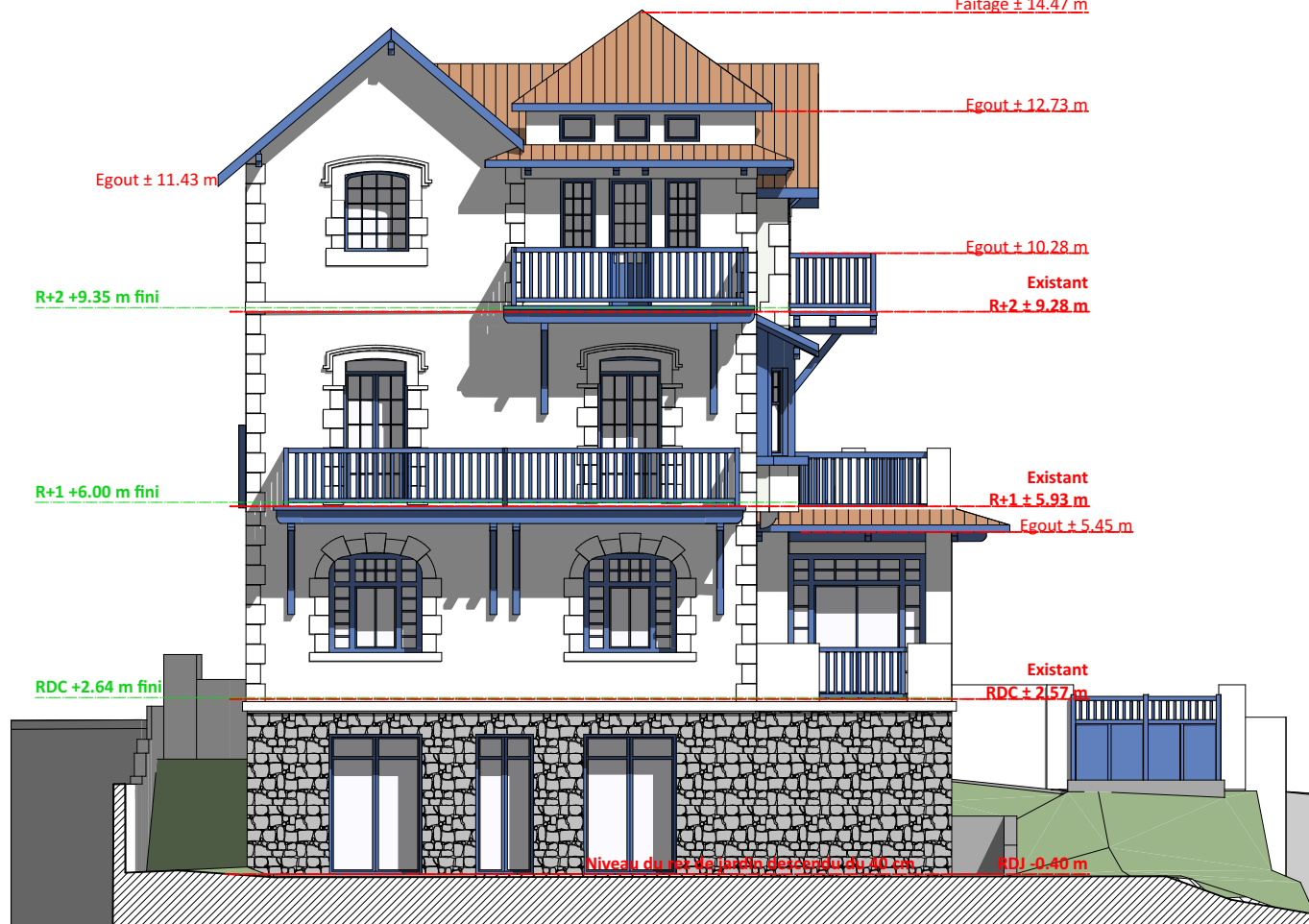
FACADE NORD - PROJET
