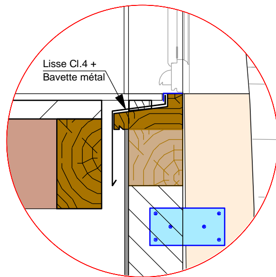
Détail seuil terrasse Ech. 1:10
