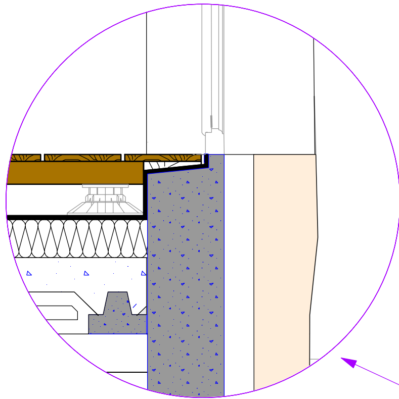
Détail seuil balcon - Ech. 1/10
