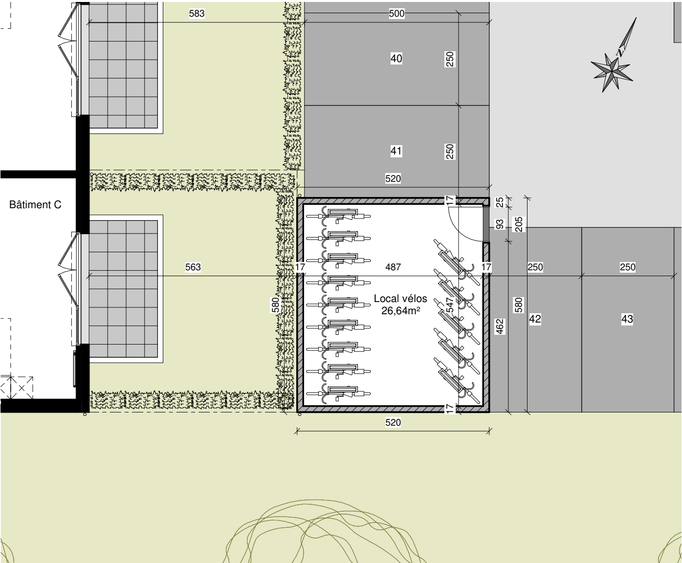
PLAN RDC Local vélos Ech : 1 : 100
