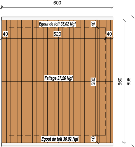
PLAN TOITURE Local vélos Ech : 1 : 100
