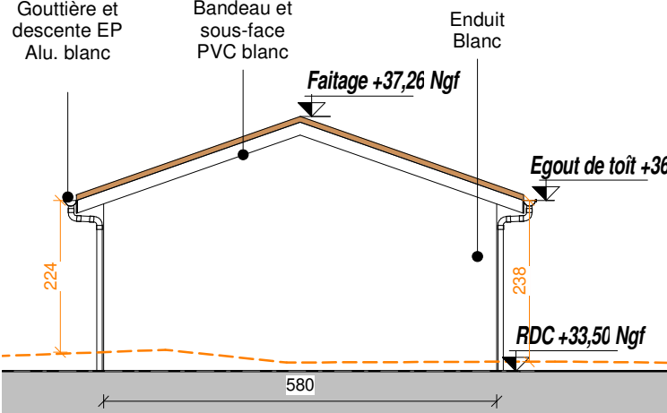
Façade Ouest Ech : 1 : 100
