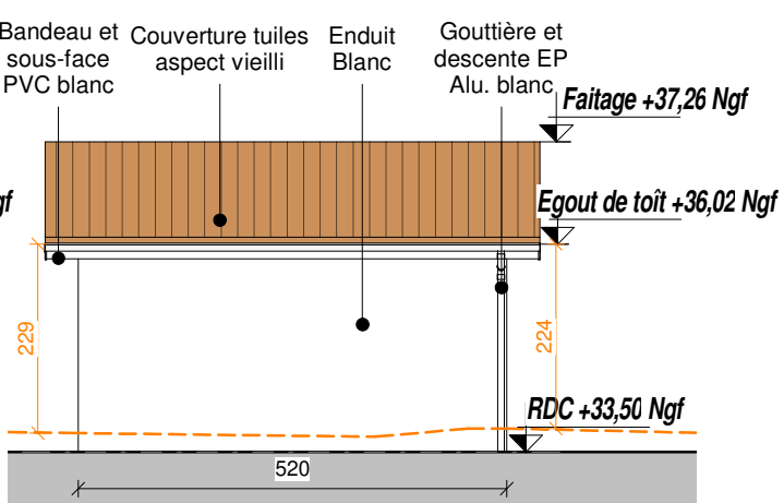
Façade Nord Ech : 1 : 100
