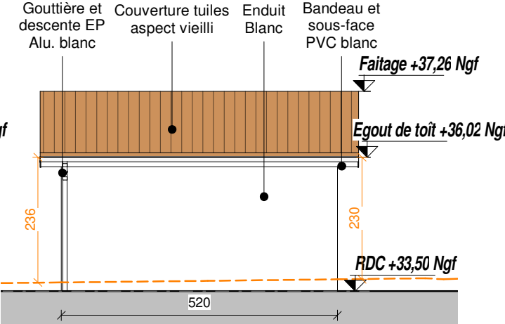
Façade Sud Ech : 1 : 100
