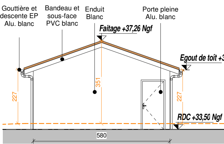
Façade Est Ech : 1 : 100
