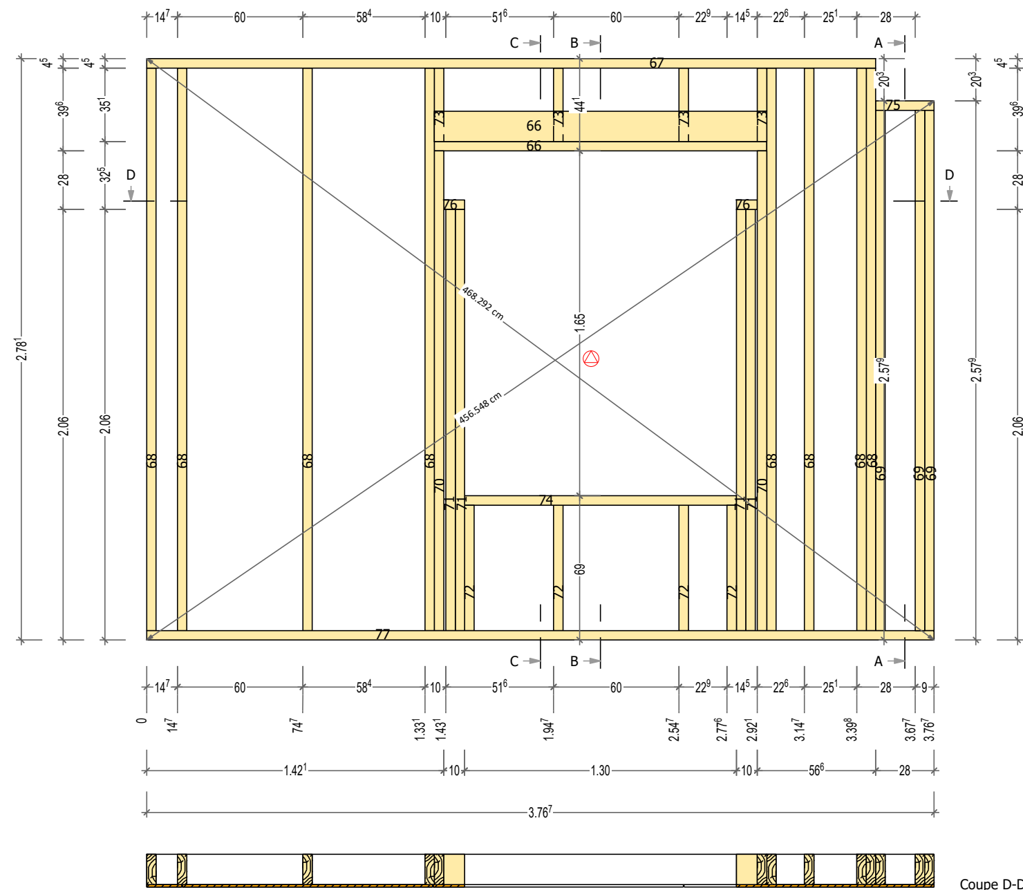
Coupe D-D
