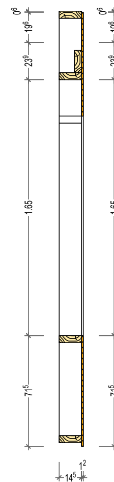
Coupe B-B
