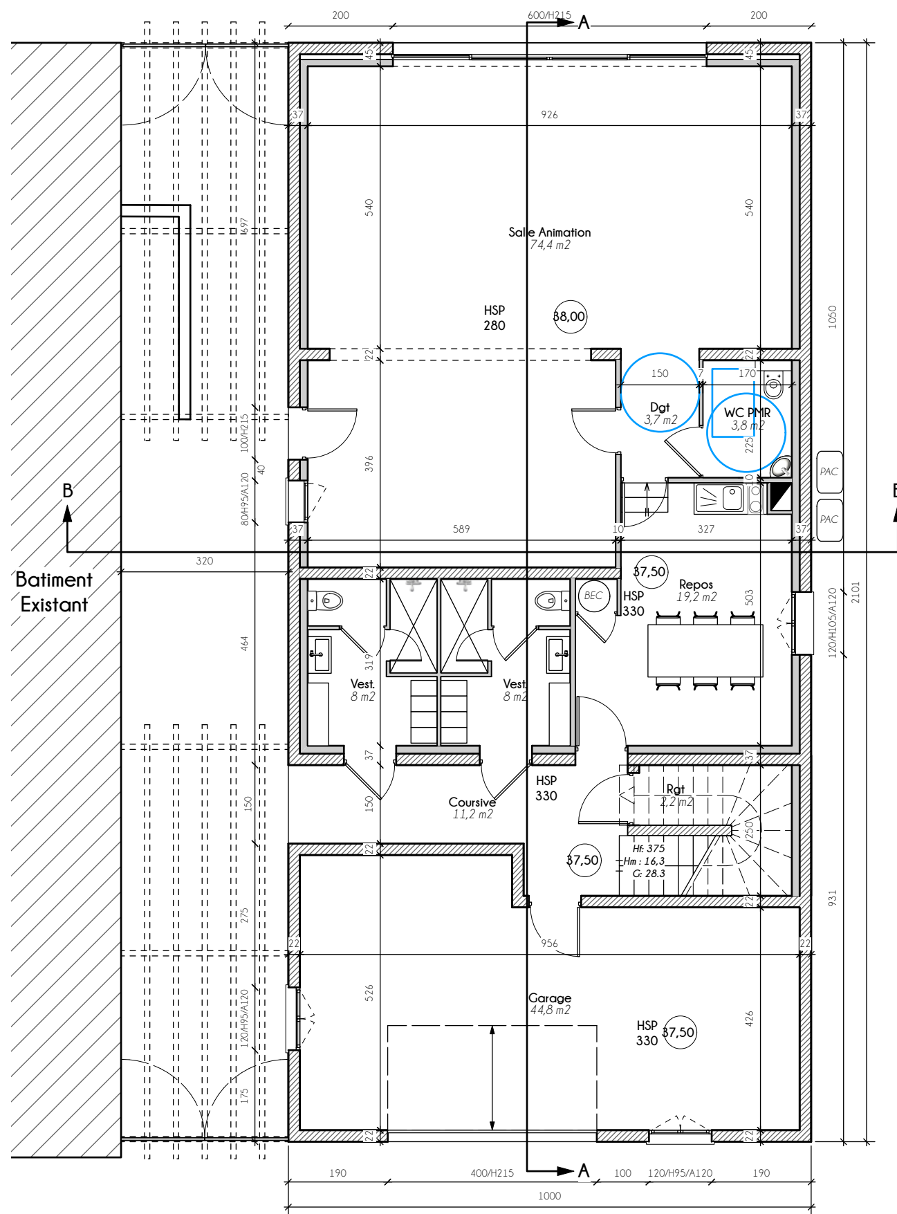
REZ-DE-CHAUSSÉE
