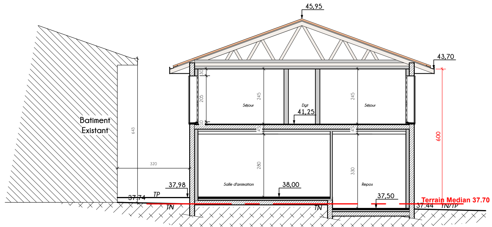
COUPE B-B
