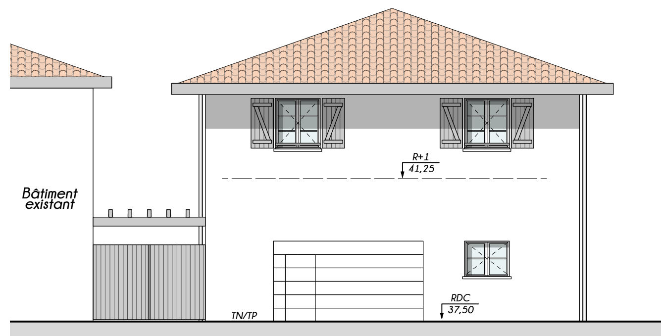
FAÇADE SUD
