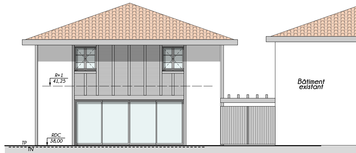
FAÇADE NORD
