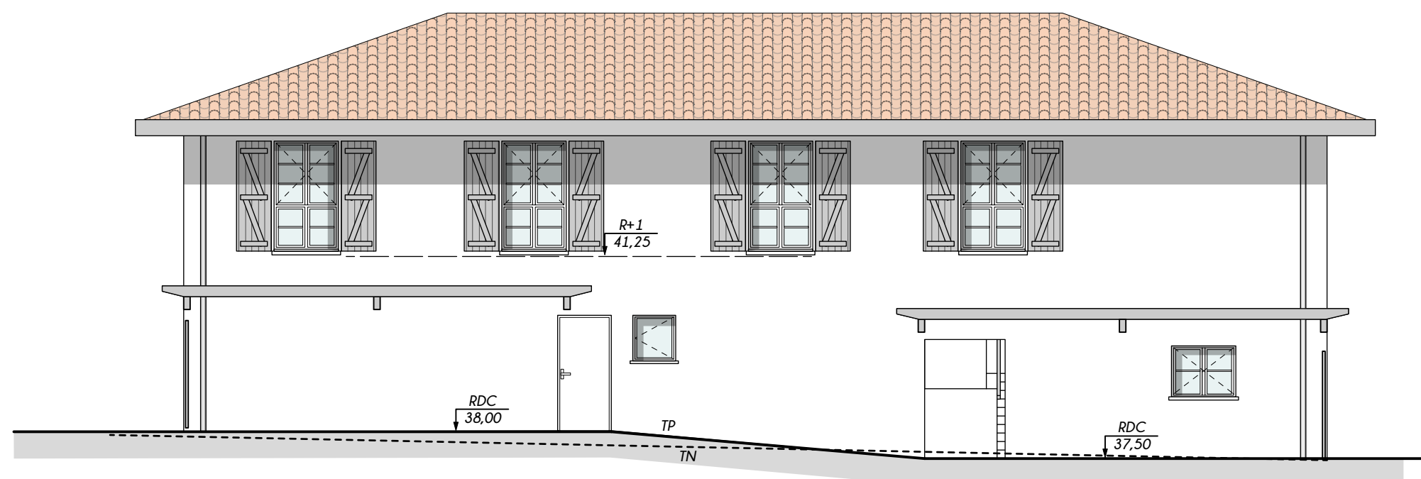
FAÇADE OUEST
